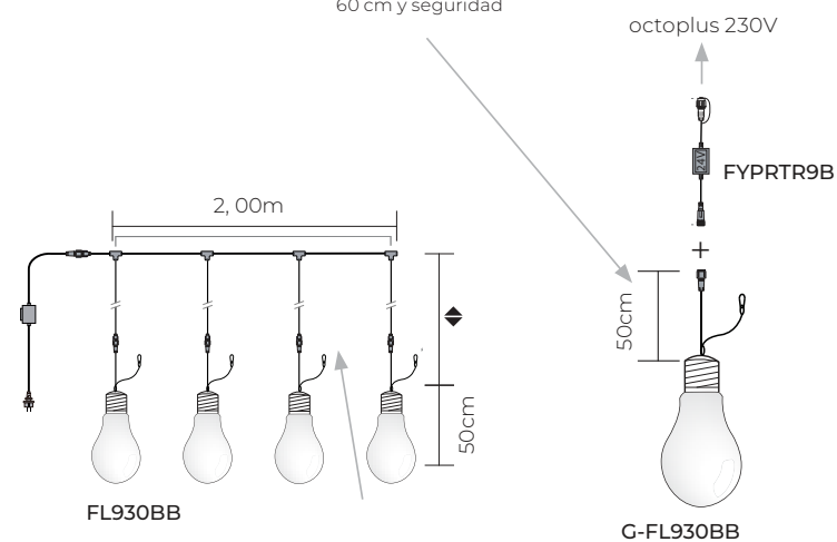
Cable de suspensión 60 cm y seguridad
